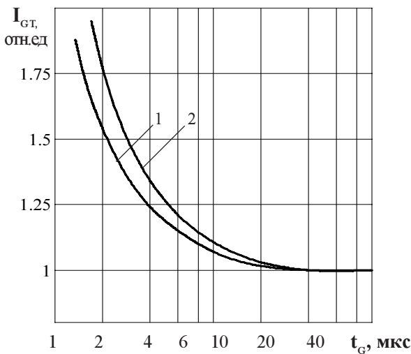
Рисунок 10 - Зависимость отпирающего импульсного тока управления I_{GT} от длительности управляющего импульса t_G при температуре перехода T_j = 25 \text{ } ^\circ\text{C} (1), T_{jmin} = \text{минус } 50 \text{ } ^\circ\text{C} (2) и напряжения в закрытом состоянии U_D = 12 \text{ В} .
