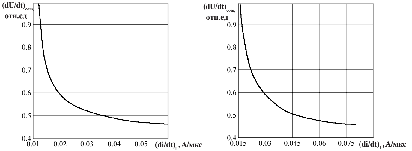
Рисунок 14 - Зависимость критической величины скорости нарастания коммутационного напряжения (dU/dt)_{com} от скорости спада предшествующего тока в открытом состоянии (di_T/dt)_f при амплитуде предшествующего тока в открытом состоянии I_T = I_{TRSM} и максимально допустимой температуре перехода T_{jн} .
