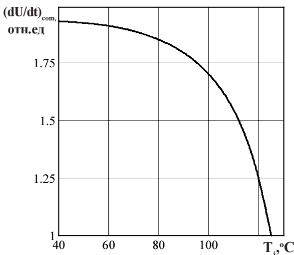
Рисунок 12 - Зависимость критической скорости нарастания коммутационного напряжения (dU_D/dt)_{com} (отн.ед.) от температуры структуры T_j = 125 \text{ } ^\circ\text{C} при I_T = I_{TRMS} , t_i = 10 \text{ мс} .
